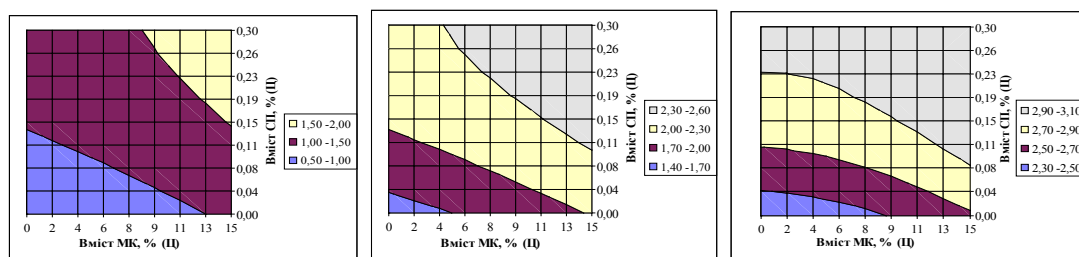
Рис. 3. Вплив СП та МК на адгезійну міцність гідроізоляційного покриття
