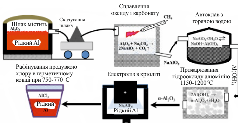
Рис. 3 . Загальна схема содового методу переробки шлаків
