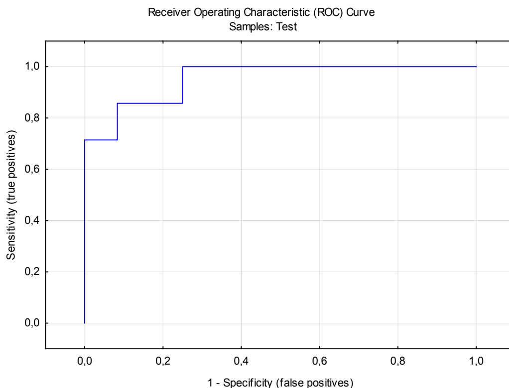
Рис. 1. ROC-крива побудованої нейронної мережі для тестової вибірки
