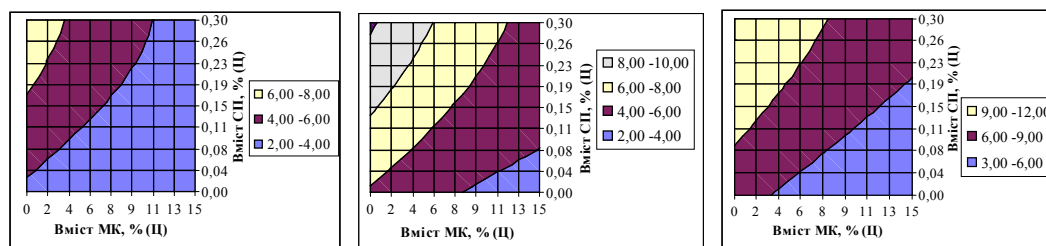
Рис. 1. Вплив СП та МК на рухомість полімерцементної суміші
