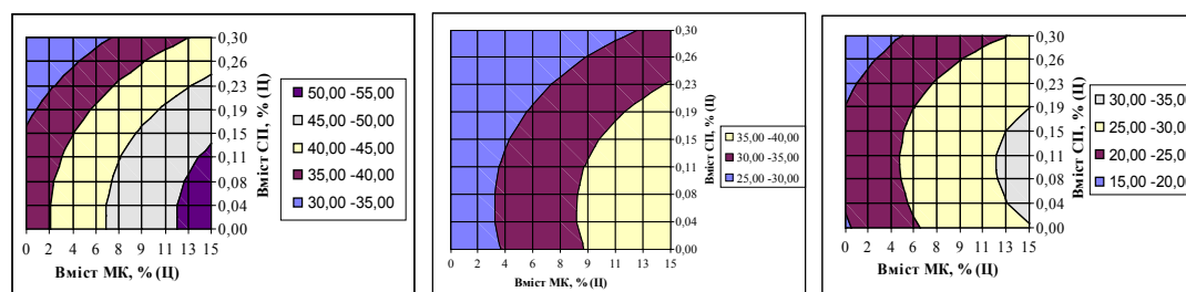
Рис. 2. Вплив СП та МК на міцність на стиск гідроізоляційного покриття
